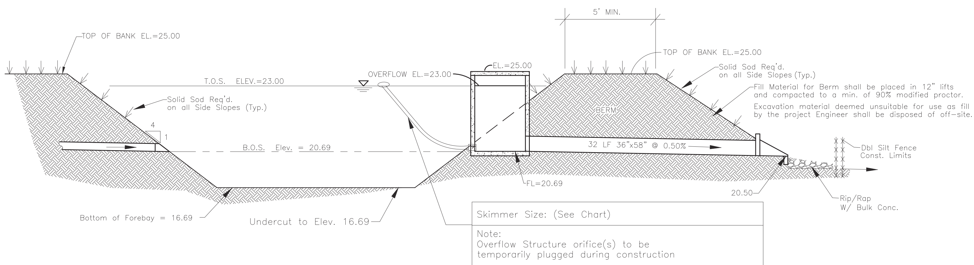
Section of Detention N.T.S.
